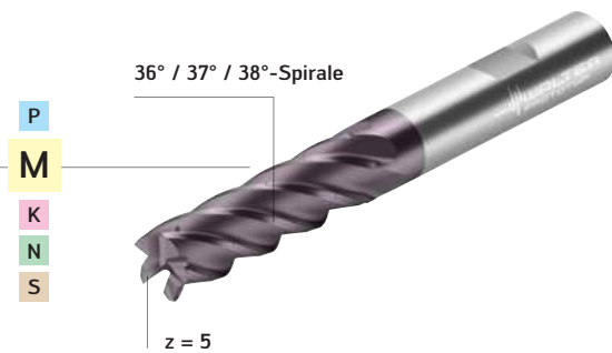
Vollhartmetallfräser Xill-tec® MC233 Advance
